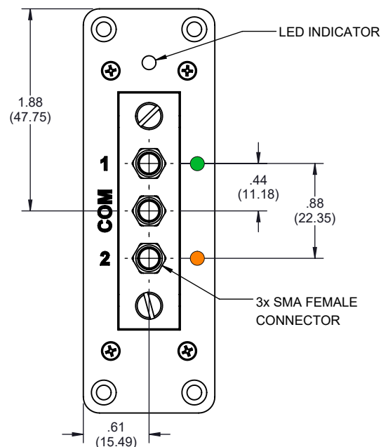
SPDTA 26GHz
