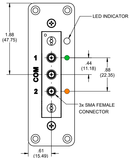
SPDTA 18GHz
