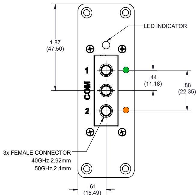
SPDT 40GHz
