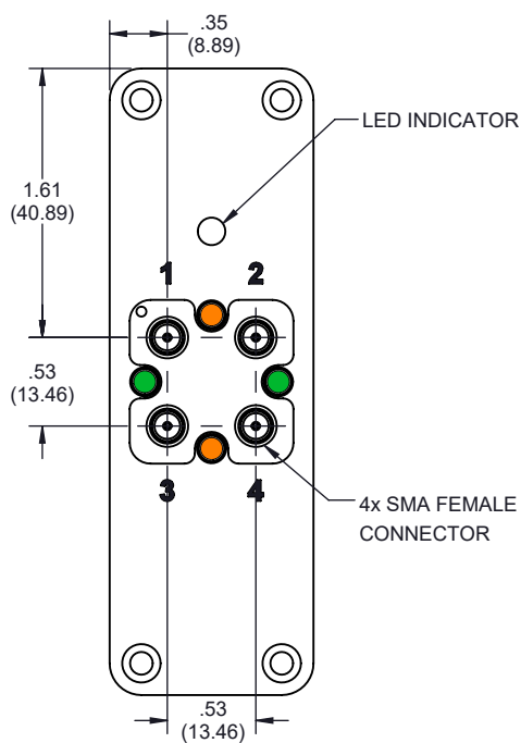
MTS 18GHz
