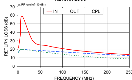
ZDC-10-1-75+ RETURN LOSS
