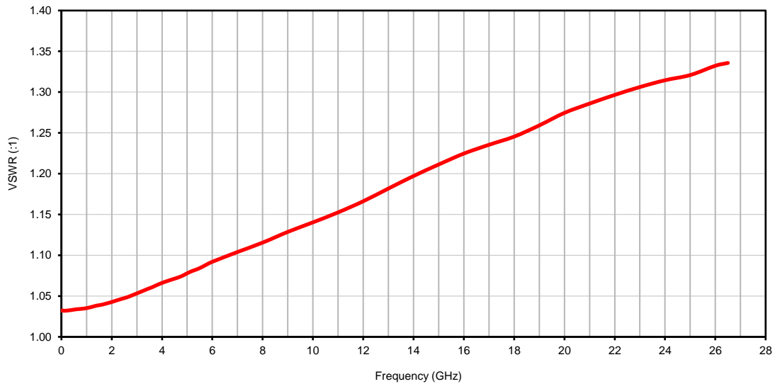
VSWR
