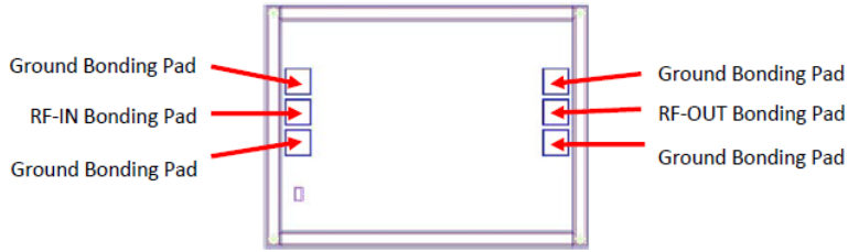
Fig 1. Die Layout
