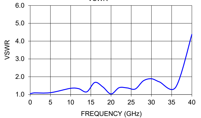
XBF-183+ VSWR
