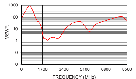
VBFZ-2340-S+ VSWR
