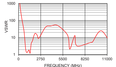
VBFZ-1065-S+ VSWR
