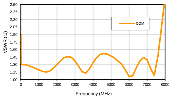
VSWR (COM)
