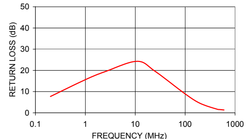
TMO-4-2+ INPUT RETURN LOSS
