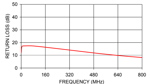
TMO-1-02+ INPUT RETURN LOSS
