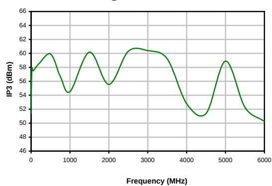
IP3 @ 0dB Attenuation
