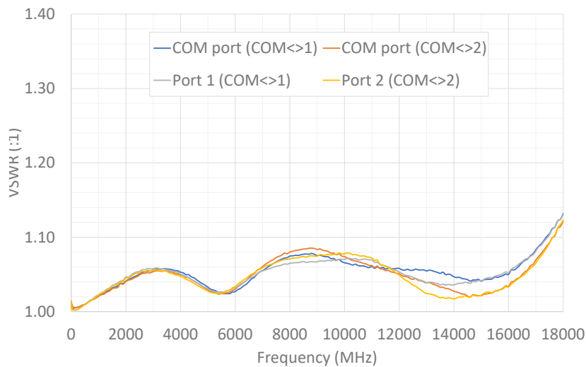
VSWR
