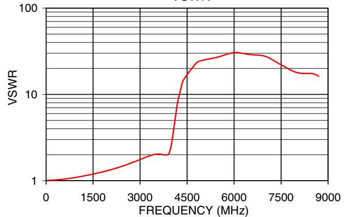
LFCN-3400D+ VSWR
