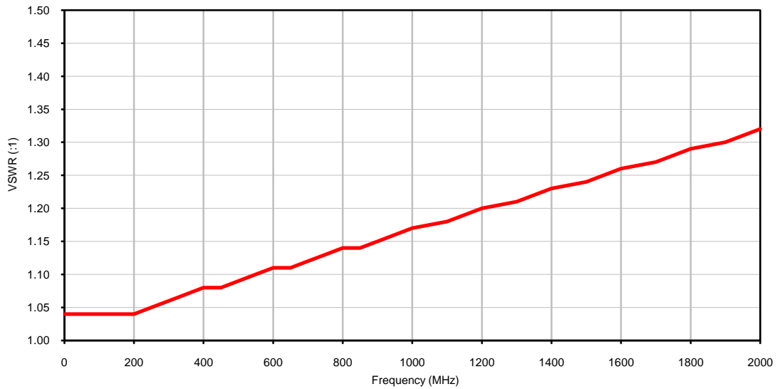
VSWR
