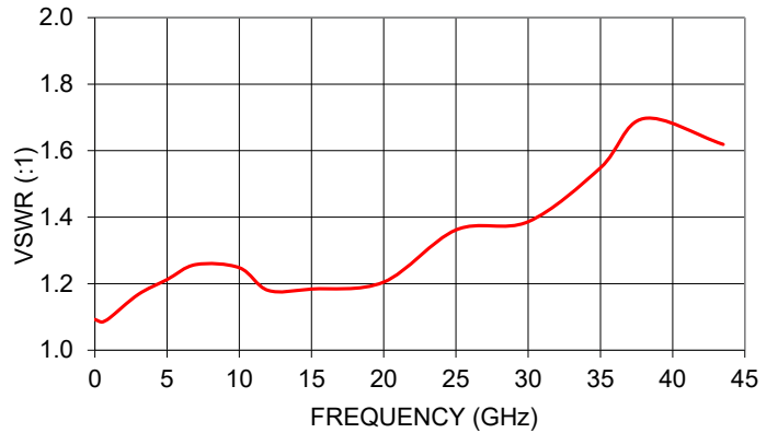
KAT-8+ VSWR
