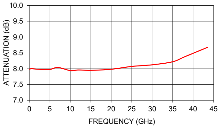
KAT-8+ ATTENUATION
