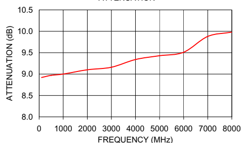
GAT-9+ ATTENUATION
