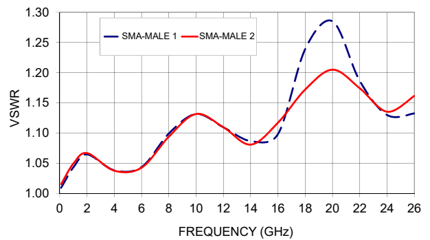
FLC-6FT-SMSM+ VSWR
