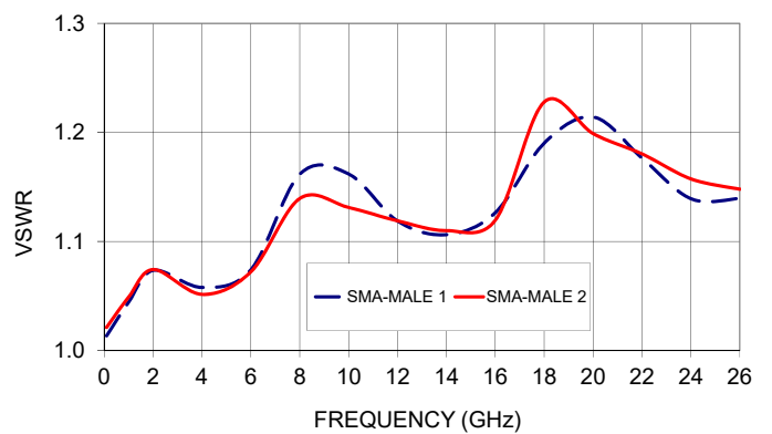
FLC-3FT-SMSM+ VSWR
