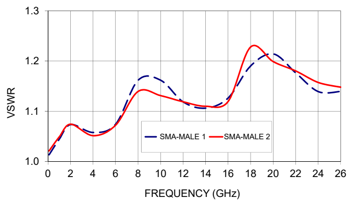
FLC-3FT-SMSM+ VSWR
