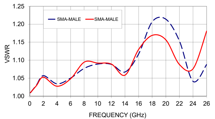
FLC-2M-SMSM+ VSWR
