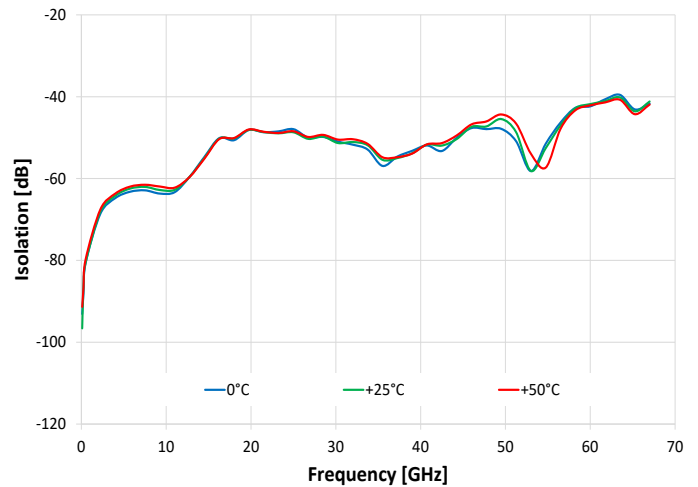
Isolation RF1 to RF2 (RF1 Active)
