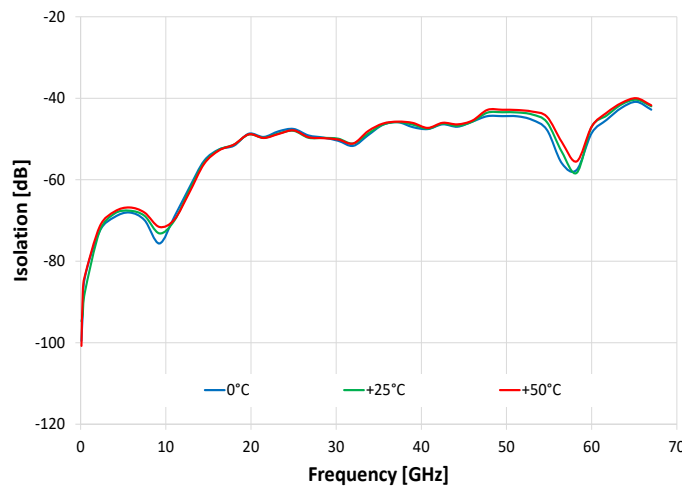
Isolation RF1 to RF2 (RF1 Active)
