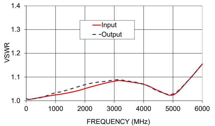
EQY-0-63+ VSWR
