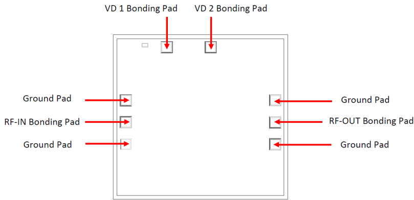
Fig 2. Die Layout
