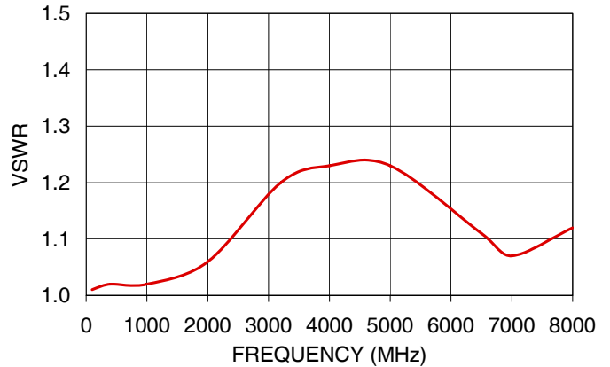
GAT-0+ VSWR
